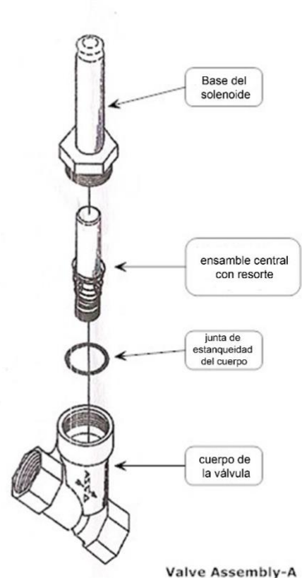
Figura 7-13: Conjunto del solenoide de la válvula
