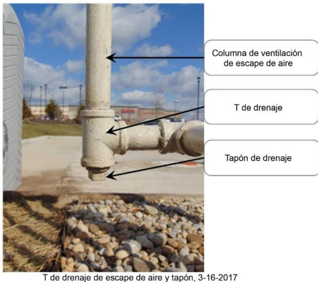
Figura 7-14: Salida de aire, conexión en T de drenaje y tapón
