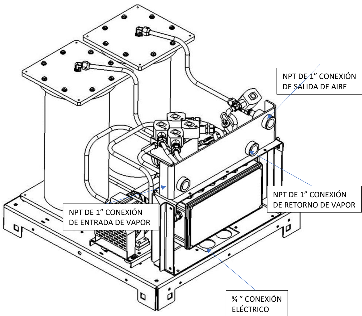
Figura 2-2: Conexiones de la GREEN MACHINE
