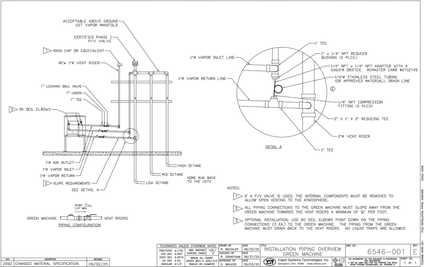
Figura 2-1: Descripción de las tuberías de vapor
