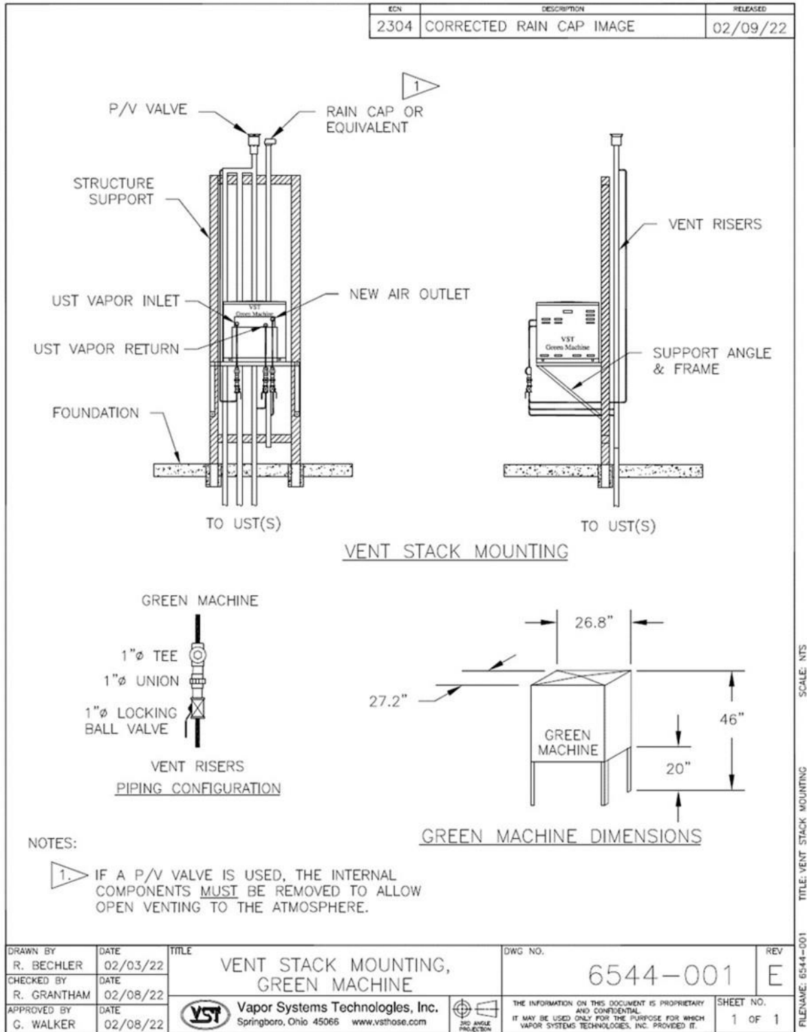
Figura 1-3: Instalación en la chimenea de ventilación
