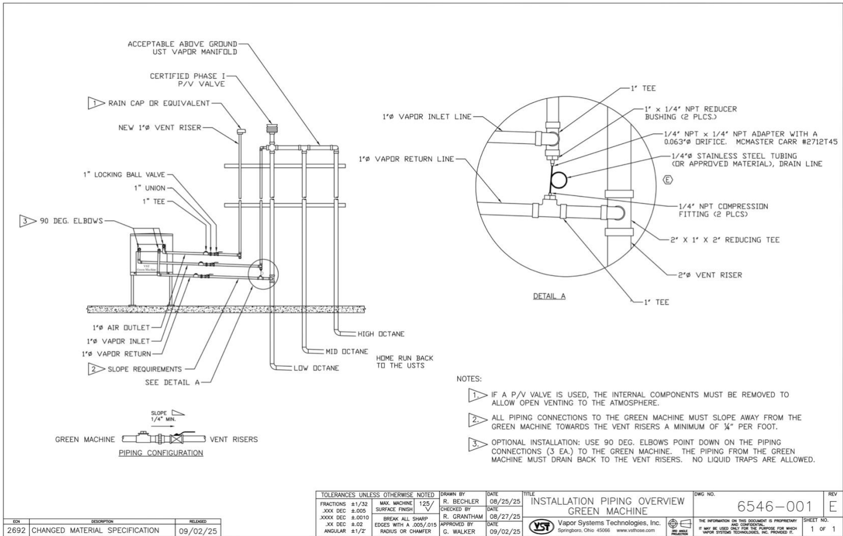
Figura 9-26: Descripción de las tuberías de vapor
