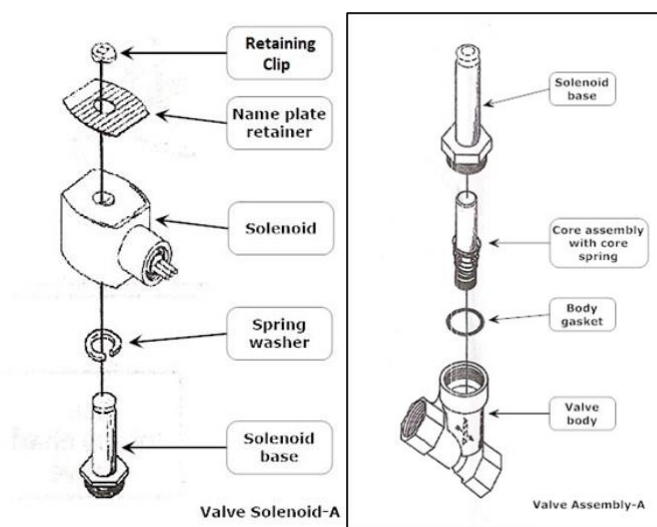
Figura 9-20: Conjunto y componentes de la válvula de control GM
