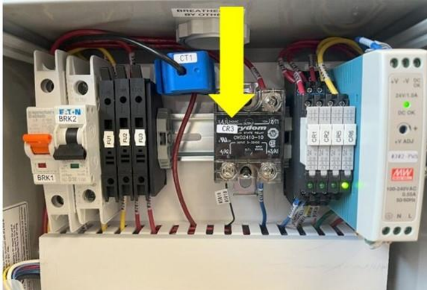
Figura 9-6: Relé de estado sólido de la bomba de vacío
