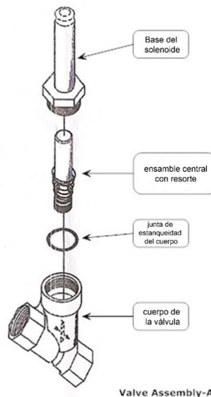
Figura 9-10: Conjunto de la válvula
