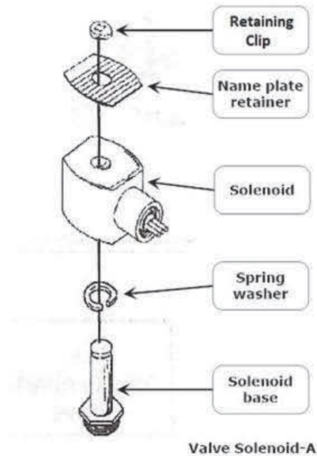
Figura 9-11: Conjunto del solenoide de la válvula
