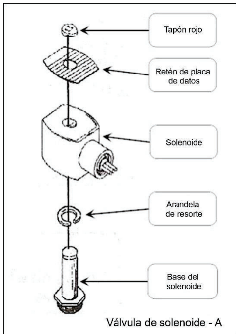
Figura 7-14: Conjunto del solenoide de la válvula
