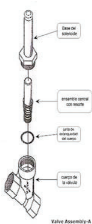
Figura 7-16: Conjunto del solenoide de la válvula
