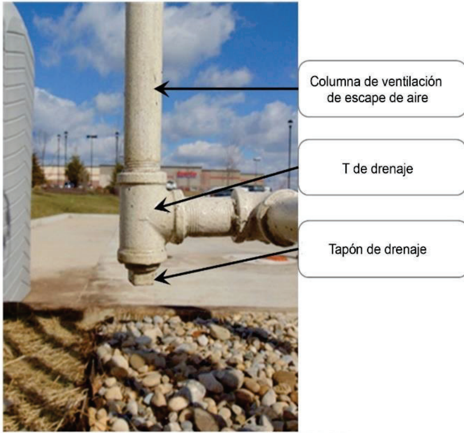
T de drenaje de escape de aire y tapón, 3-16-2017
