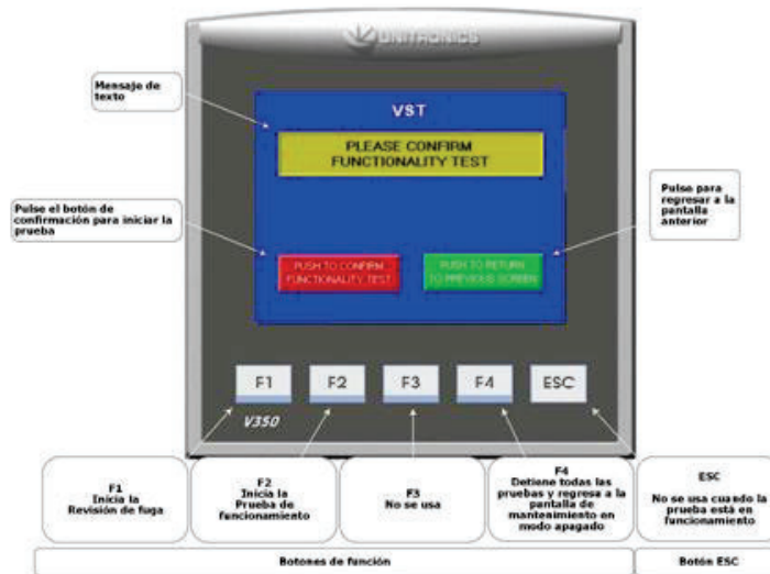
Figura 7-6: Botón de confirmación de la prueba de funcionamiento
