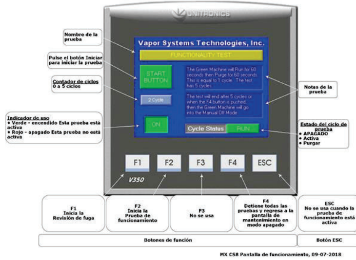
Figura 7-5: Pantalla de prueba de funcionamiento
