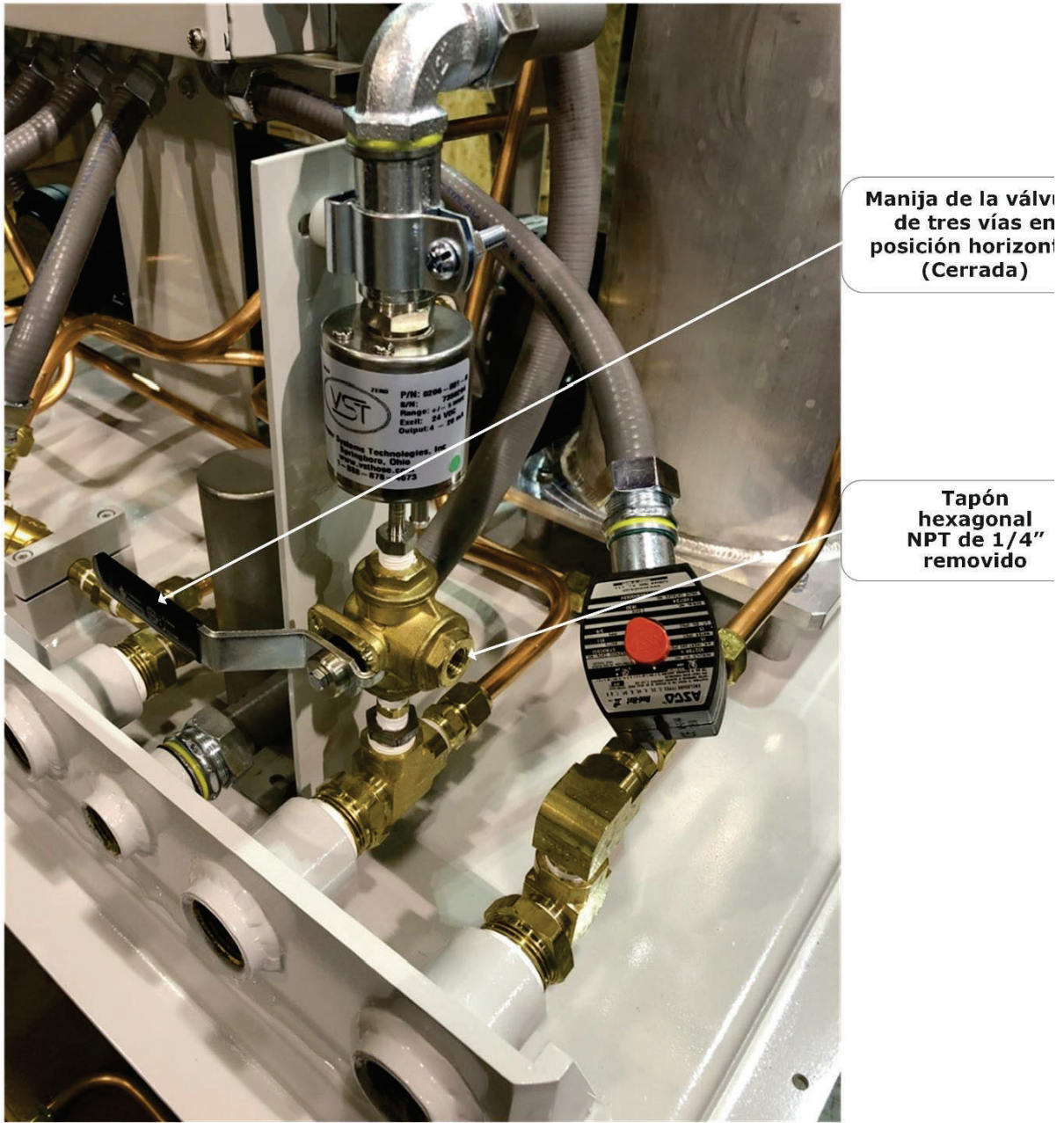
Prueba 2 de verificación del sensor de presión de la GM CS8, 17/6/2018
