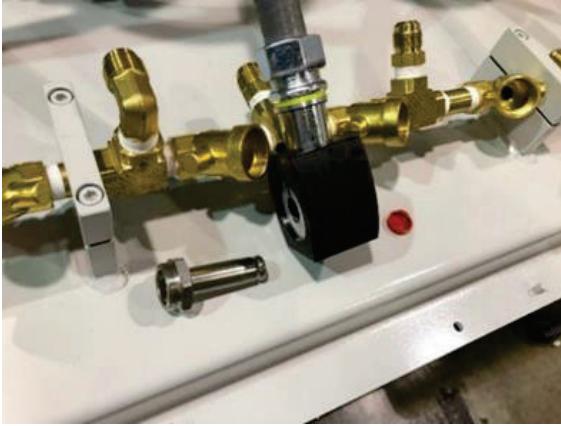
Figura 9-29: Solenoides con base del solenoide y tapón rojo
