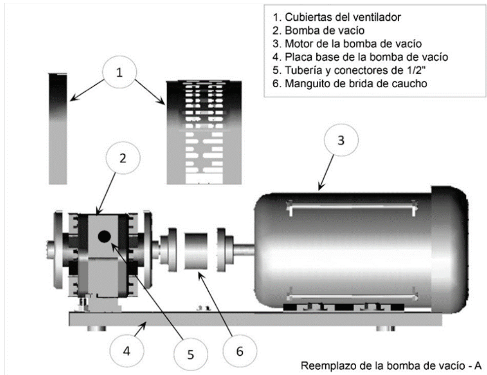
Figura 9-21: Componentes de la bomba de vacío
