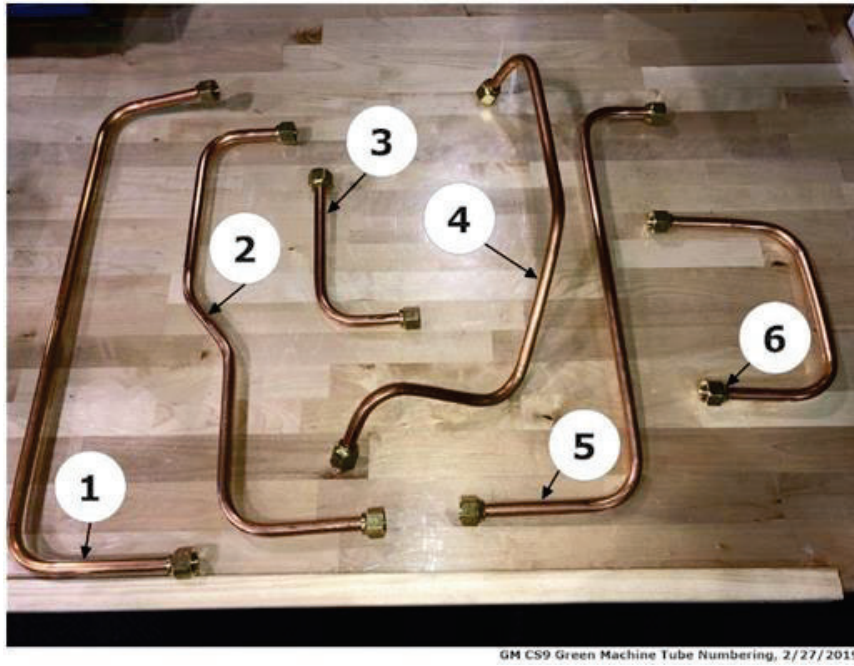
Figura 9-23: Tuberías 1 a 6 retiradas
