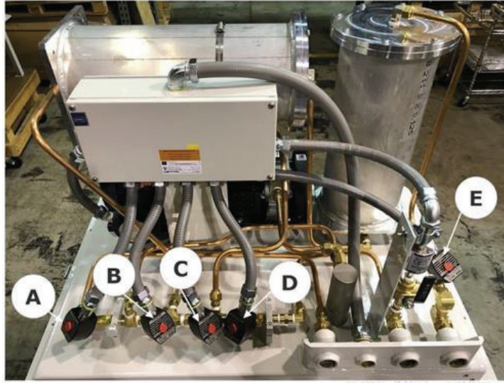
Válvulas del colector de la GM CS9. 28/2/19
