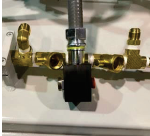
Figura 9-30: Solenoides con base del solenoide y tapón rojo instalados
