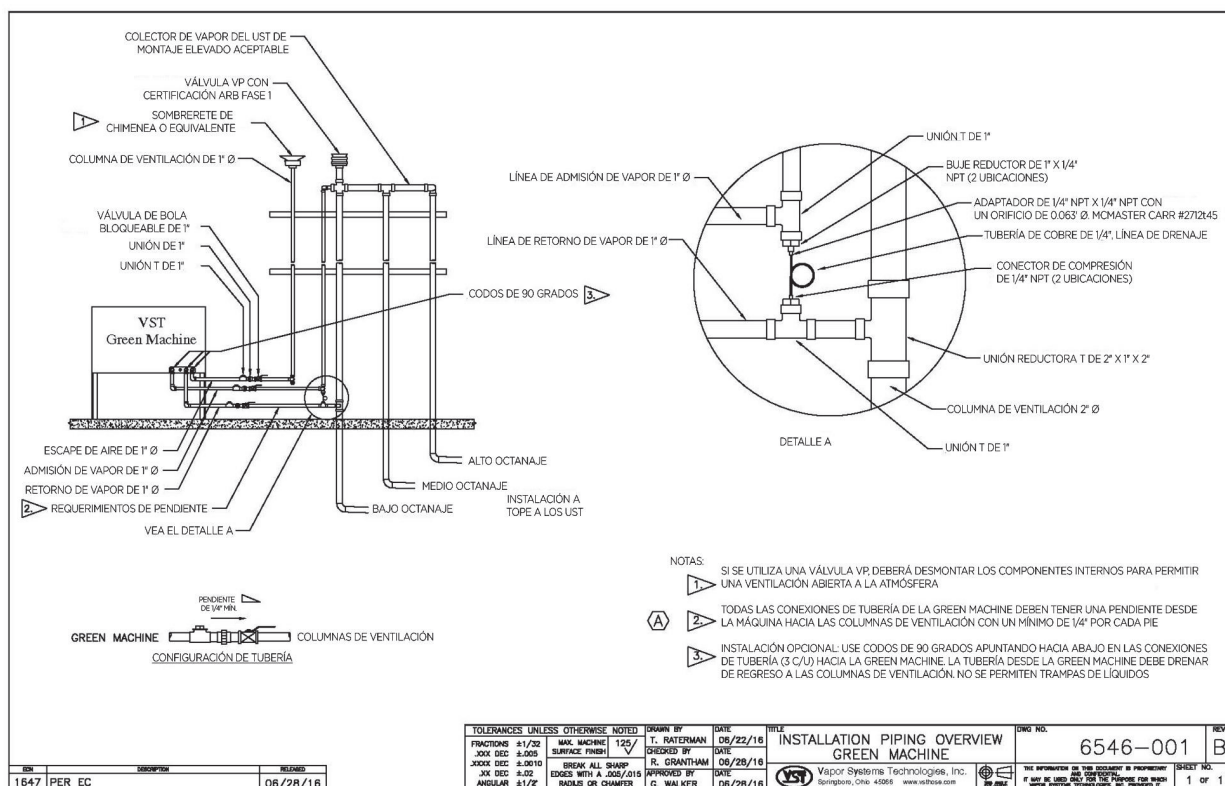
Figura 6-2: Descripción de las tuberías de vapor
