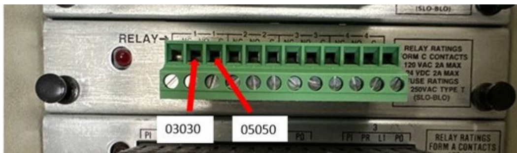
Figure 3-2: Relé de salida Veeder-Root TLS-350
