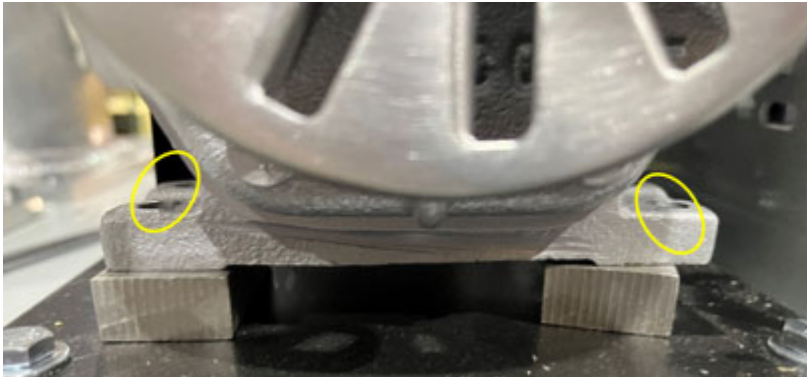
Figure 9-11: Retire los 4 pernos de montaje del motor de la placa base del motor
