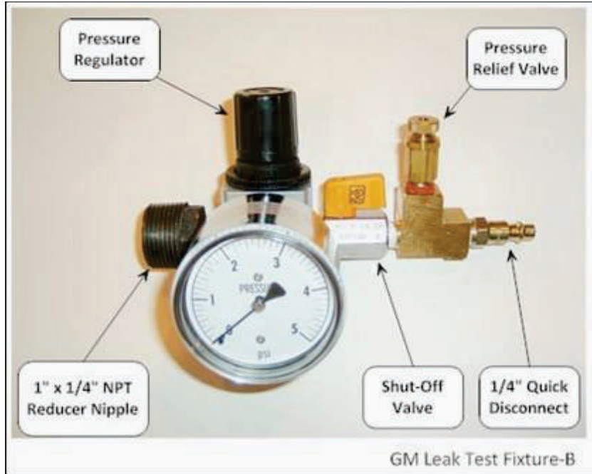
Figura 9-28: Dispositivo para revisión de fugas
