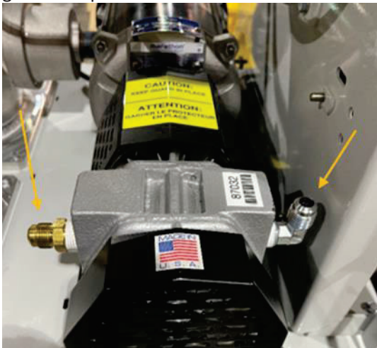
Figura 9-15: Retire los conectores de bronce de la tubería de ambos lados de la bomba de vacío
