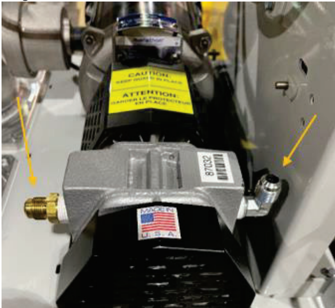
Figura 9-7: Retire los dos tubos en la bomba
