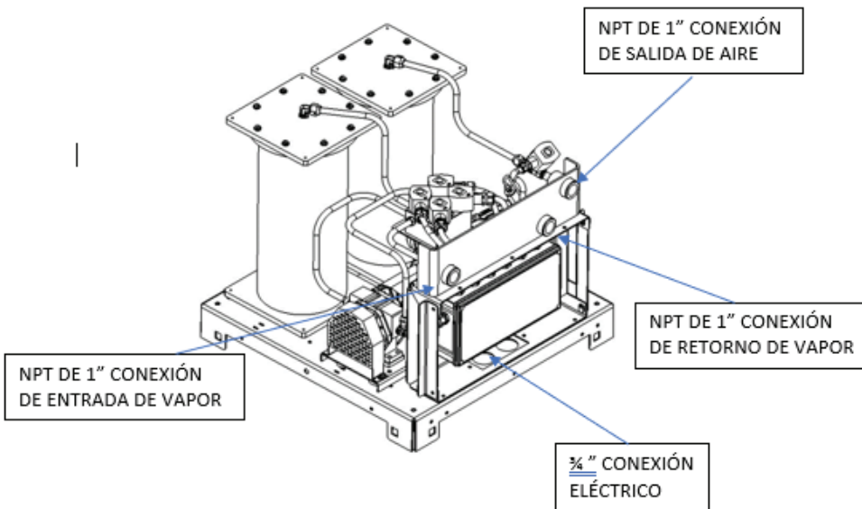
Figure 7-7: Diagrama de operación de la GREEN MACHINE
