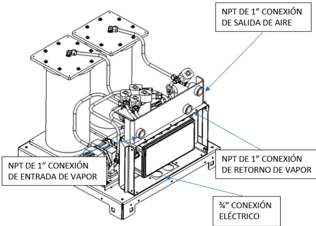
Figure 6-6: Diagrama de funcionamiento GREEN MACHINE
