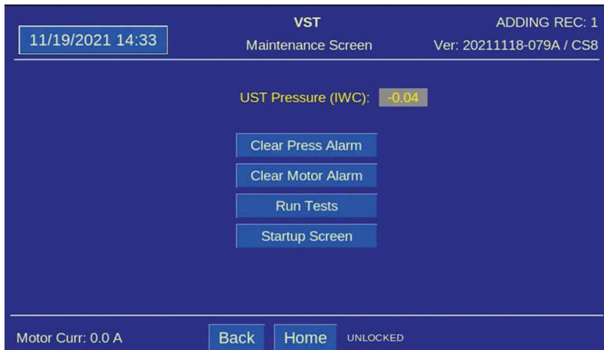
Figure 6-2: Pantalla de mantenimiento
