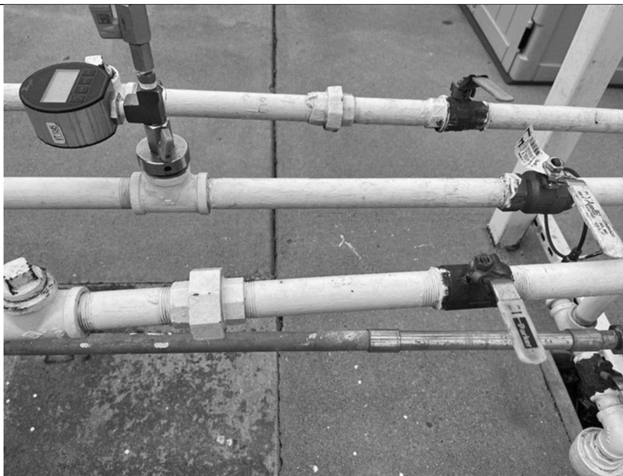
Figure 9-29: GREEN MACHINE con las tuberías de ingreso y retorno de vapor y salida de aire
