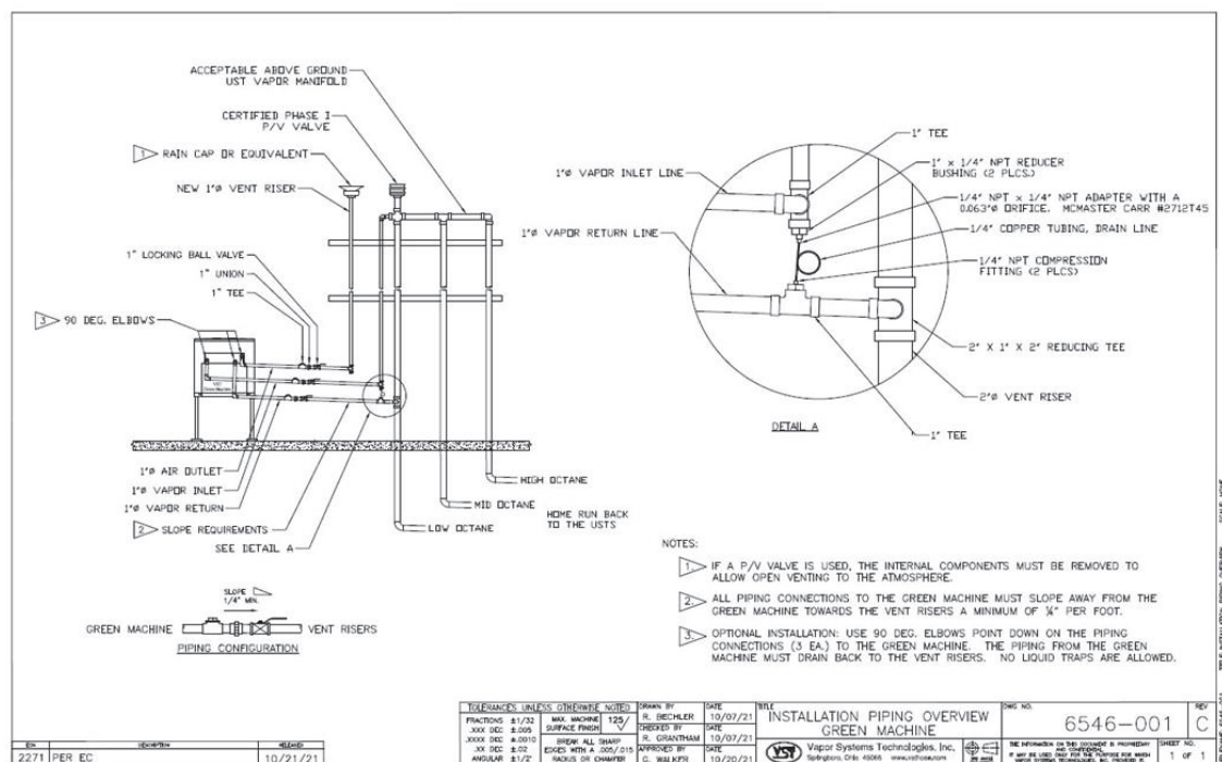
Figure 6-3: Esquema de la tubería de vapores de la GREEN MACHINE
