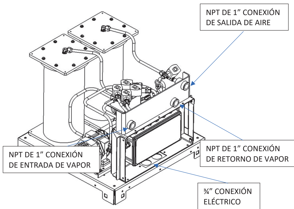
Figure 6-6: Diagrama de funcionamiento GREEN MACHINE
