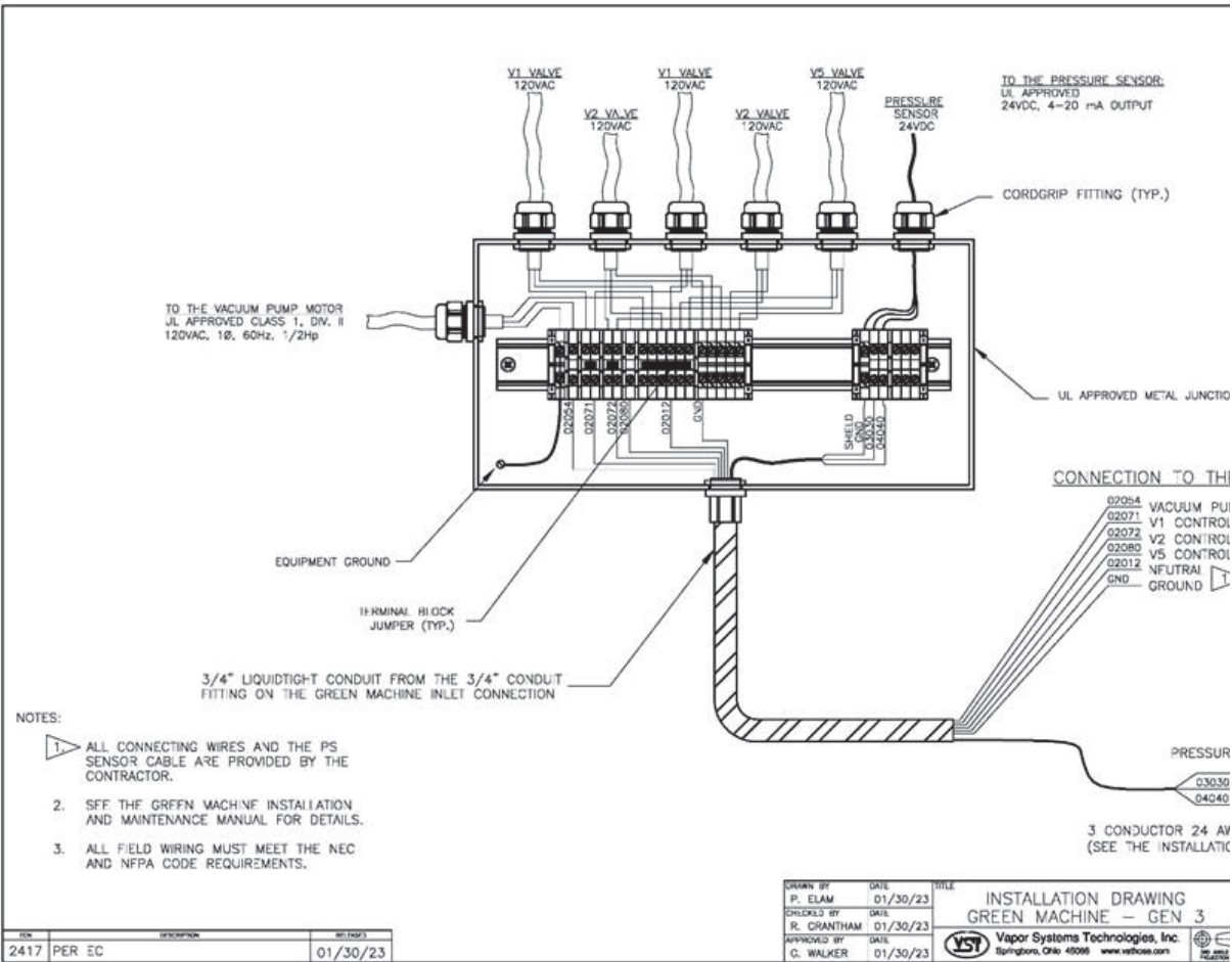
Figure 3-7: Cableado de campo de la caja de conexiones internas del GREEN MACHINE
