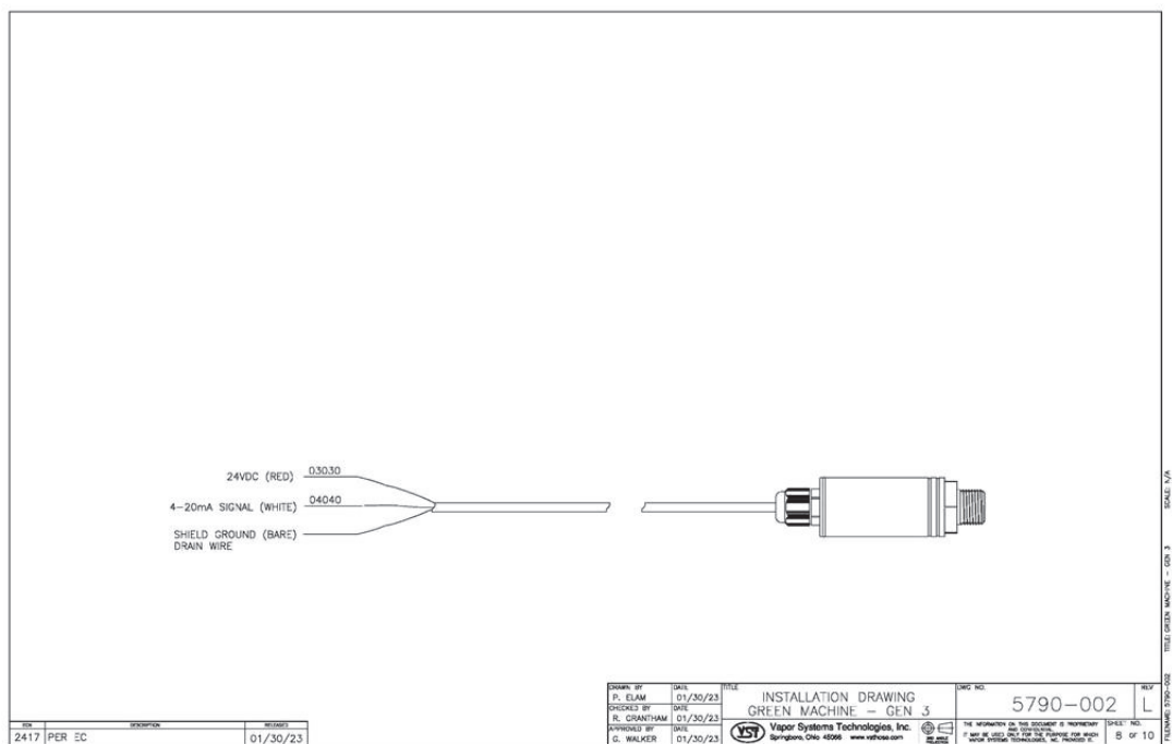
Figure 3 8: Diagrama de cableado del sensor de presión
