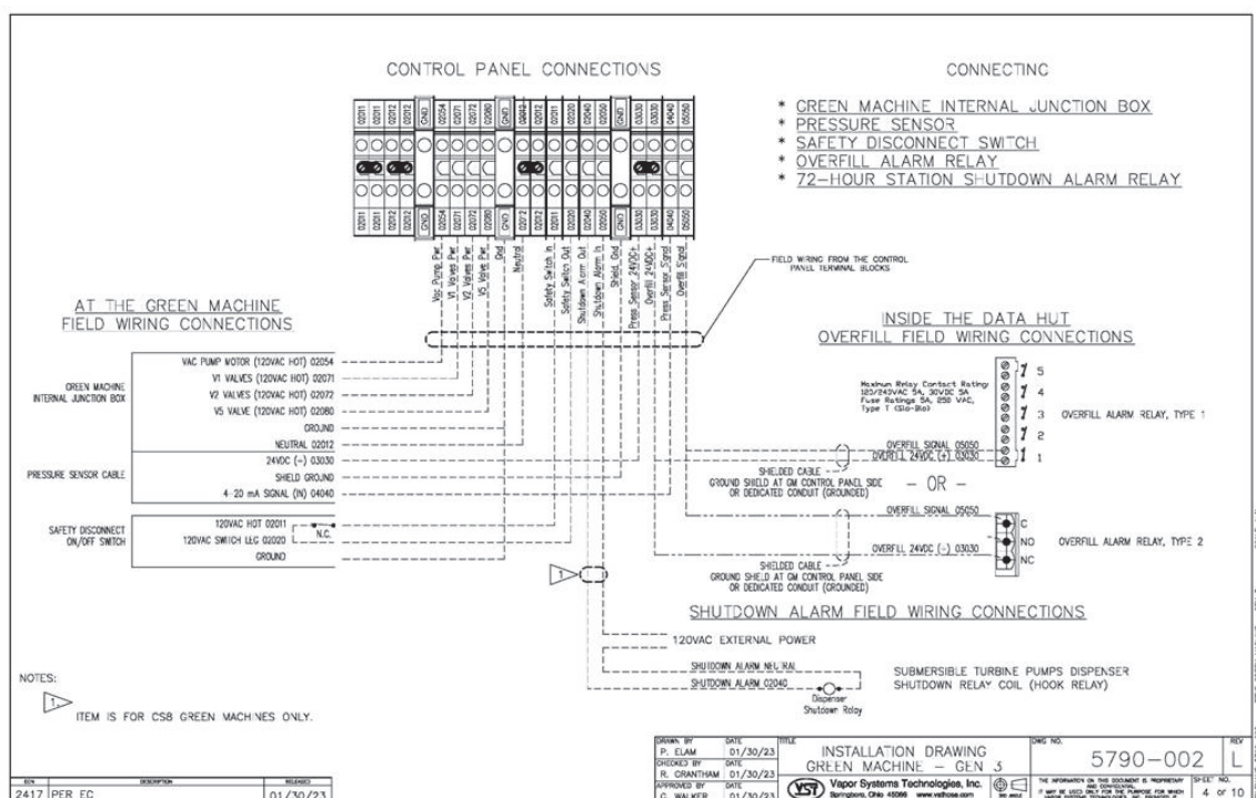
Figure 3-6: Cableado de campo del panel de control de VST
