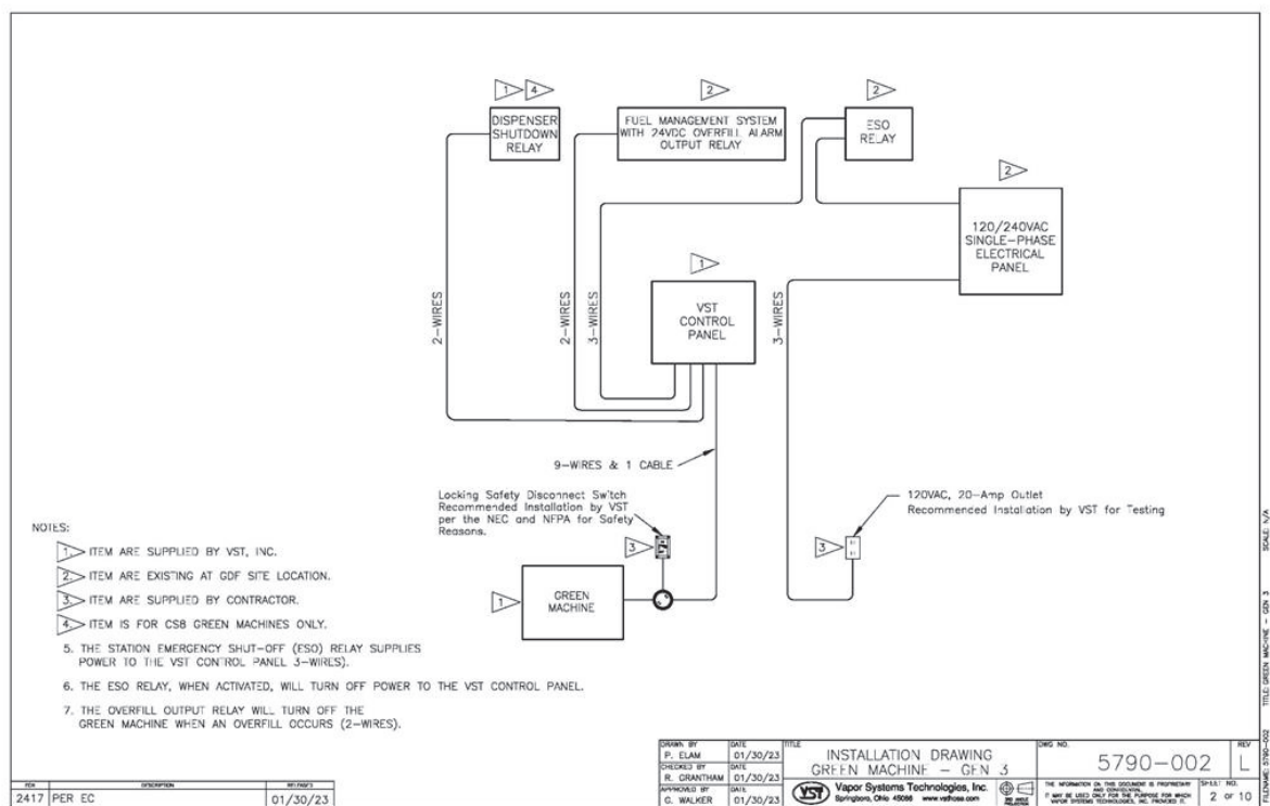
Figure 3-4: Descripción de la instalación de la GREEN MACHINE
