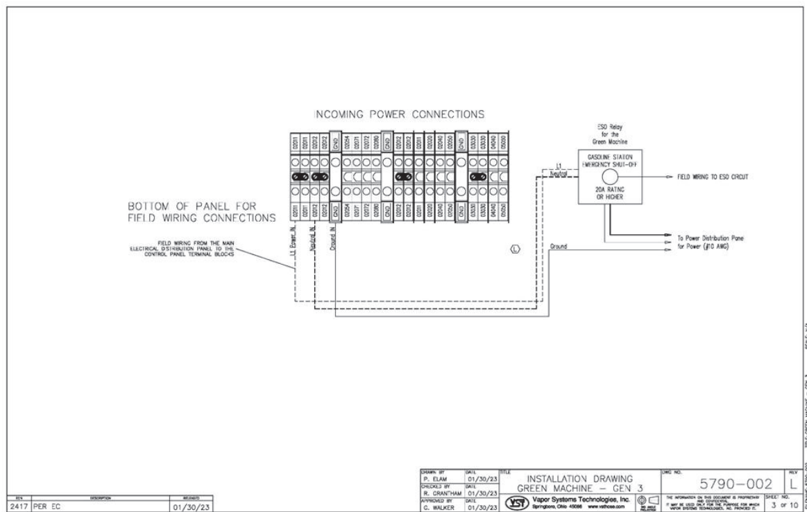
Figure 3-5: Conexiones de energía del panel de control de VST
