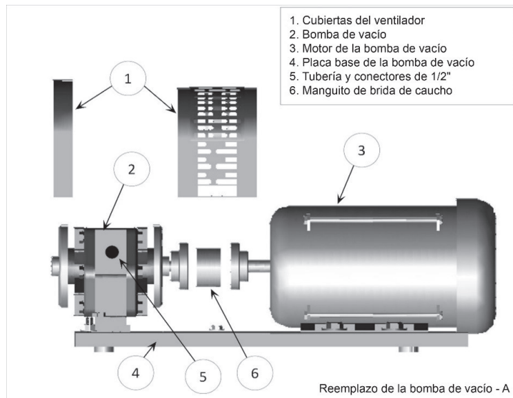
Figura: 9.16 Componentes de la bomba de vacío
