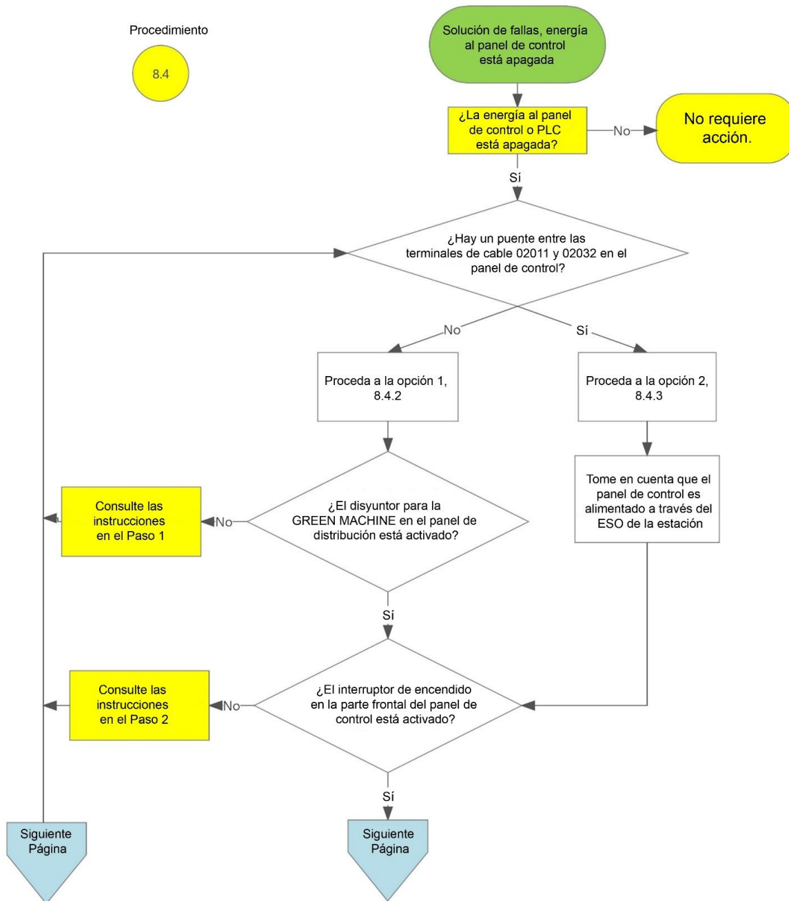
Figura: 8.5 Alimentación al panel de control de VST o al controlador está desconectada
