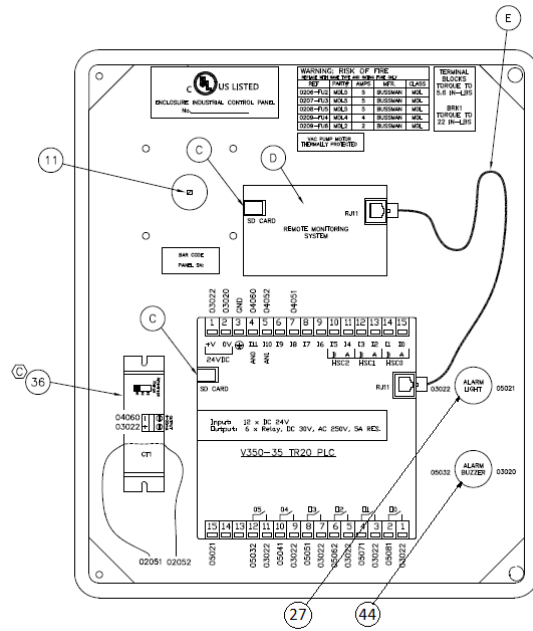
Figura: 9.3 Panel de control de VST, Piezas de repuesto del interior de la cubierta delantera
