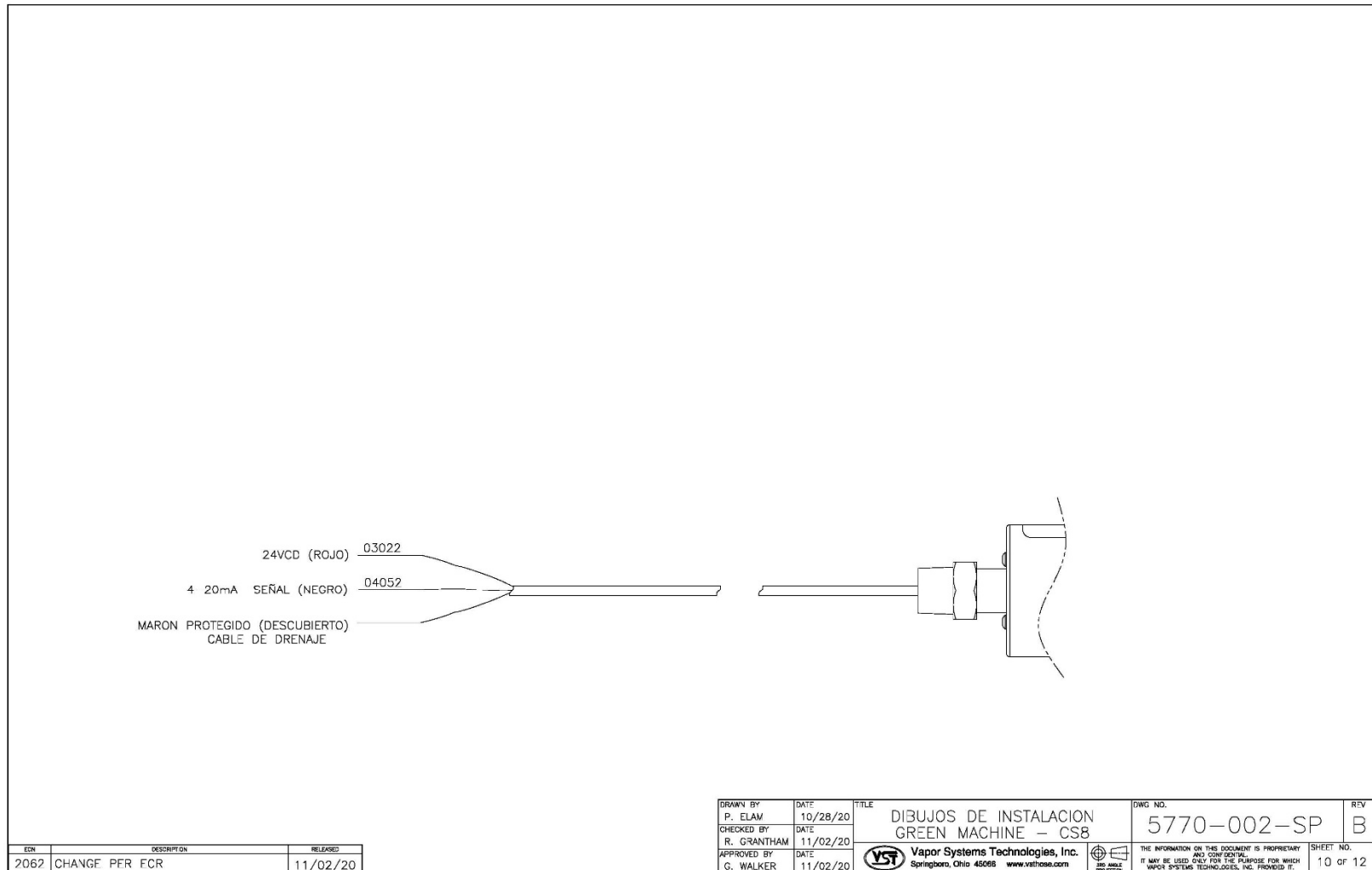
Figura: 3.11 Diagrama de cableado del sensor de presión
