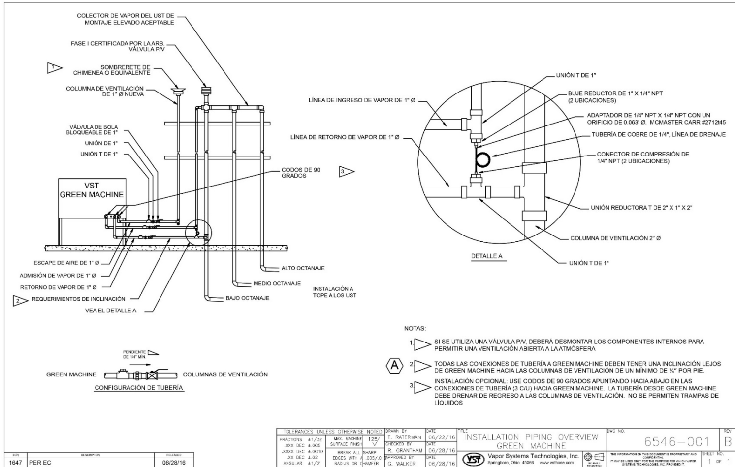
Figura: 6.2 Descripción de las tuberías de vapor
