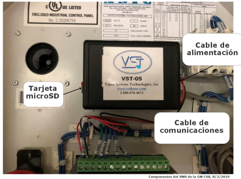
Figura: 9.11 Componentes del RMS
