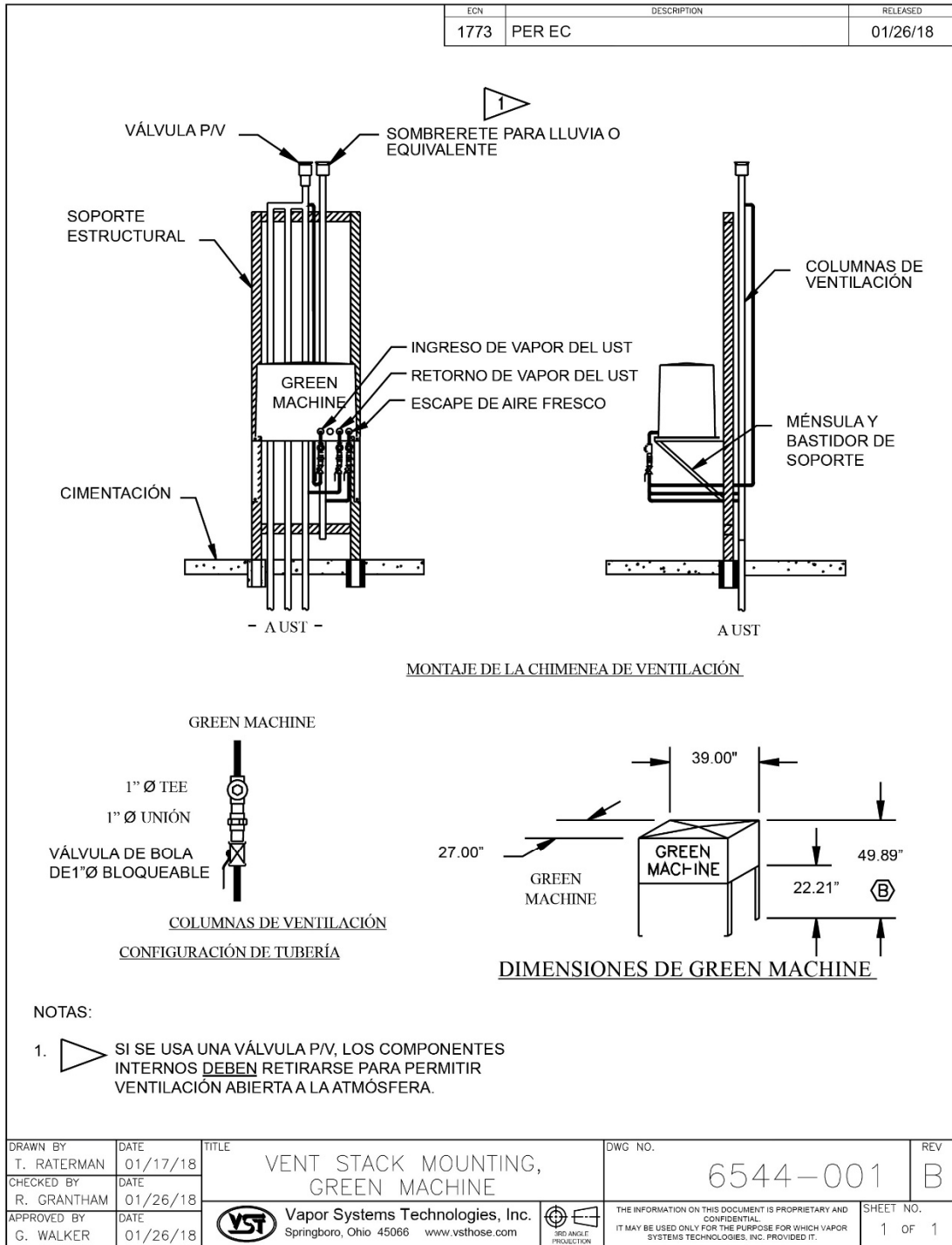
Figura: 1.4 Instalación en la chimenea de ventilación
