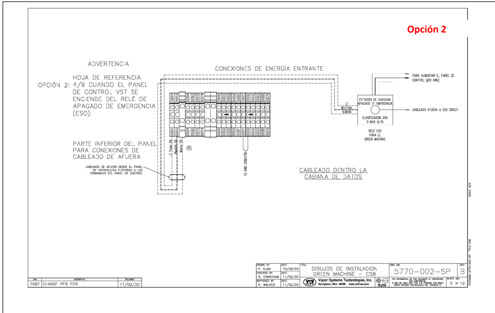
Figura: 8.9 Plano de la instalación eléctrica
