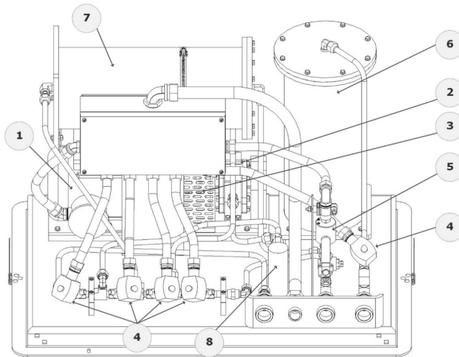
Numeración de las piezas de la GM CS8, 17/6/2019
