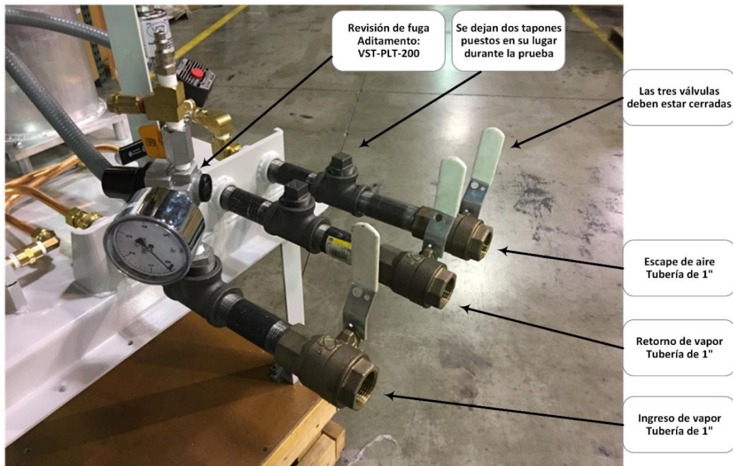
Aditamento de prueba de fugas GM - B, 11-2-2016
