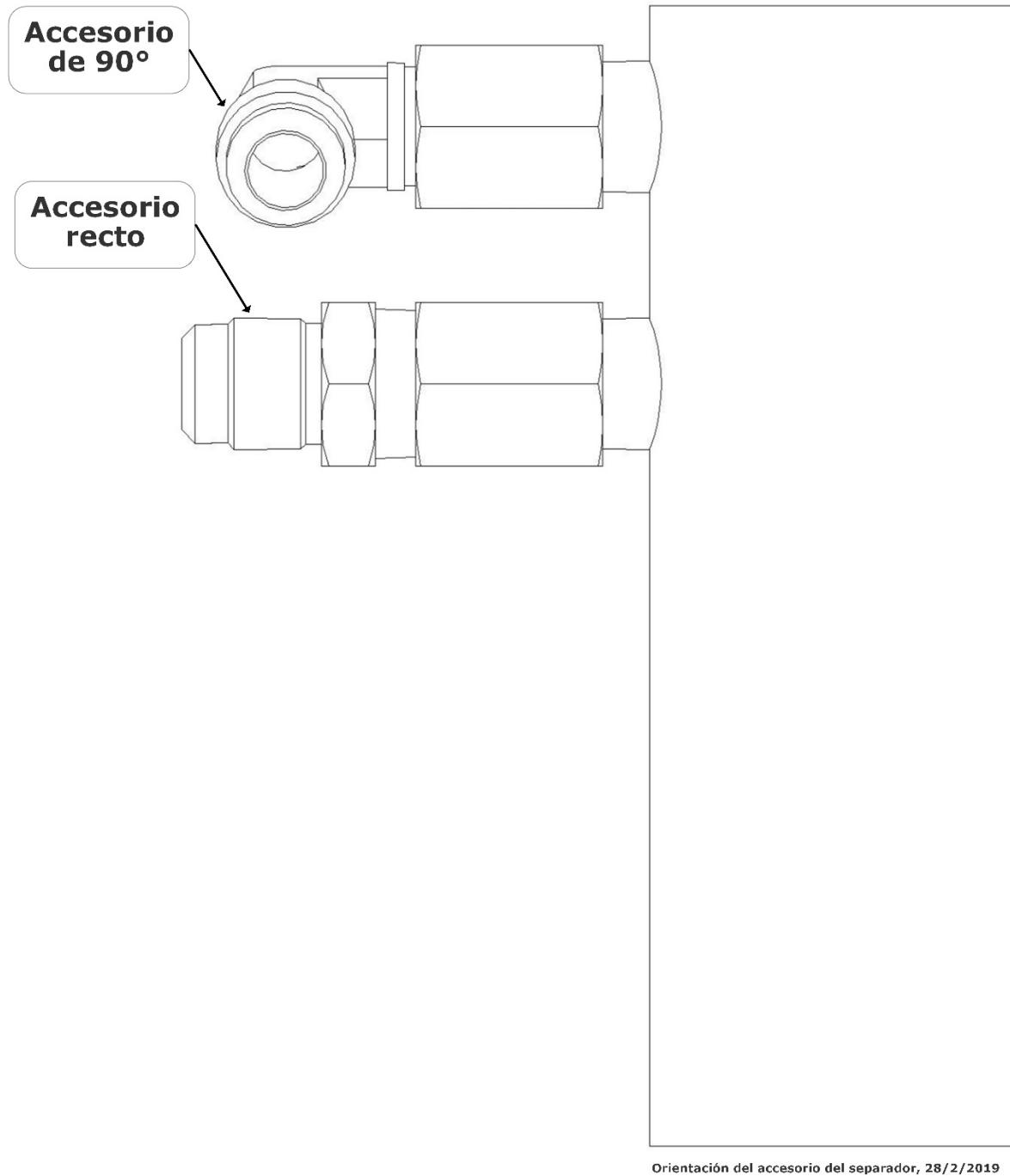
Figura: 7.19 Orientación del accesorio del separador
