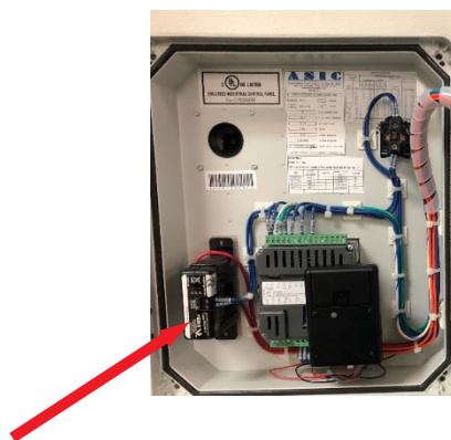
Figura: 5.6 Ubicación del dispositivo de almacenamiento de respaldo
