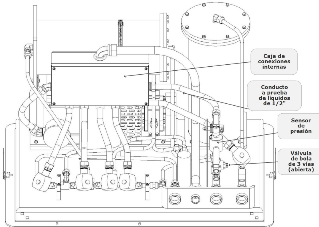
Reemplazo del sensor de presión de la GM CS8, 17/6/2019
