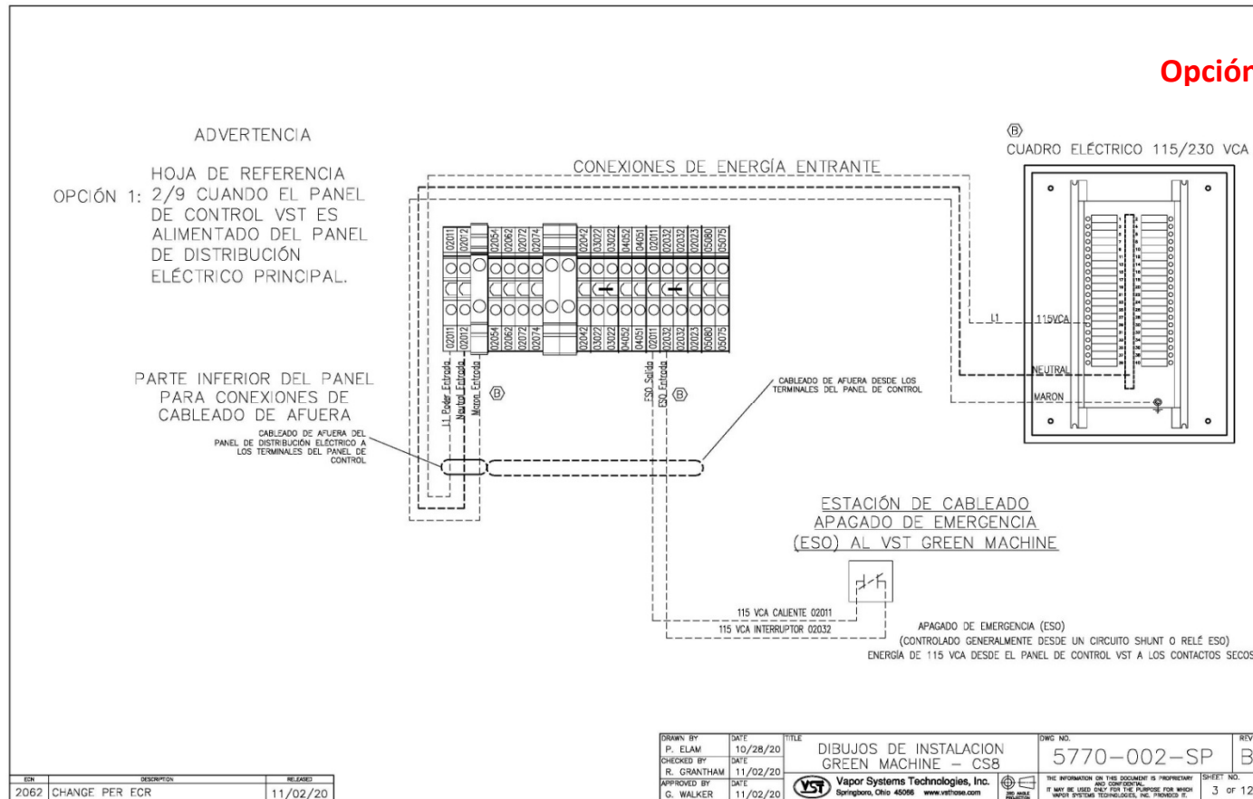
Figura: 8.7 Conexiones entrantes de energía
