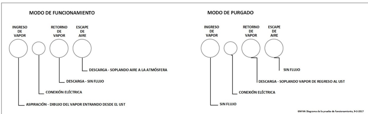
Figura: 6.10 Diagrama de operación de la GREEN MACHINE
