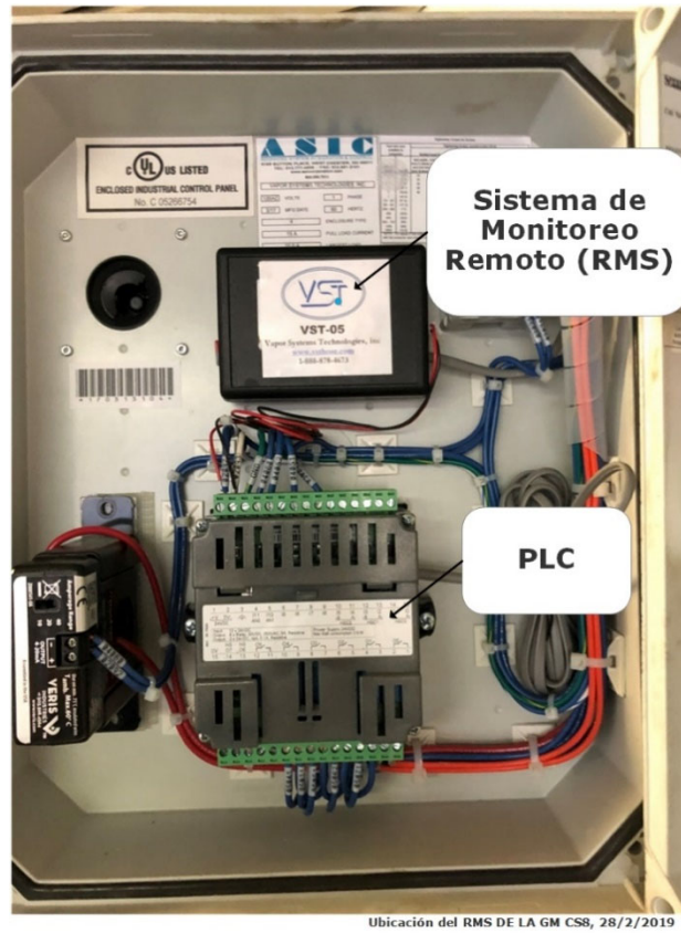
Figura: 9.10 Ubicación del RMS
