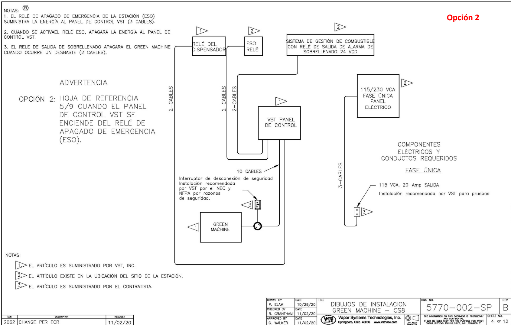
Figura: 3.5 Descripción de la instalación de la GREEN MACHINE - Opción 2
