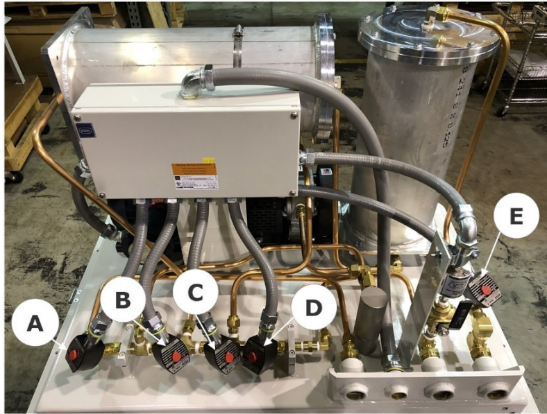
Válvulas del colector de la GM CS9. 28/2/19 Figura: 9.25 Válvulas del colector
