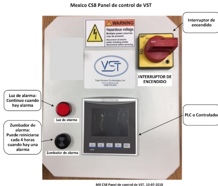
Figura: 4.1 Panel de control México CS8 de VST, vista frontal
