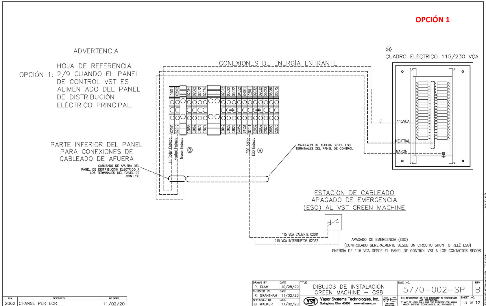
Figura: 3.4 Conexiones de ESO y alimentación de energía del panel de control de VST - Opción 1
