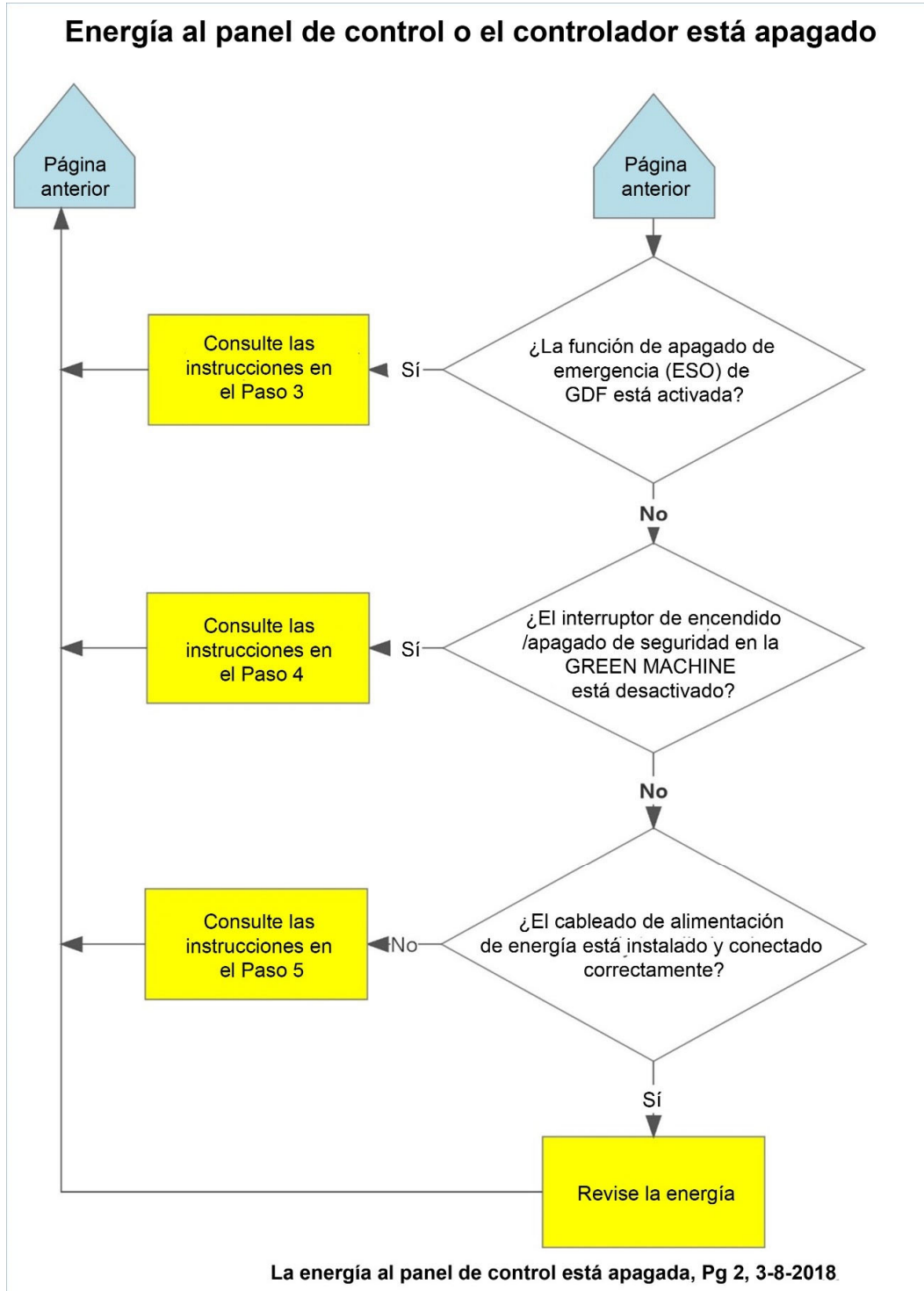
Figura 8-5 (continuación) Alimentación al panel de control de VST o al controlador está desconectada
