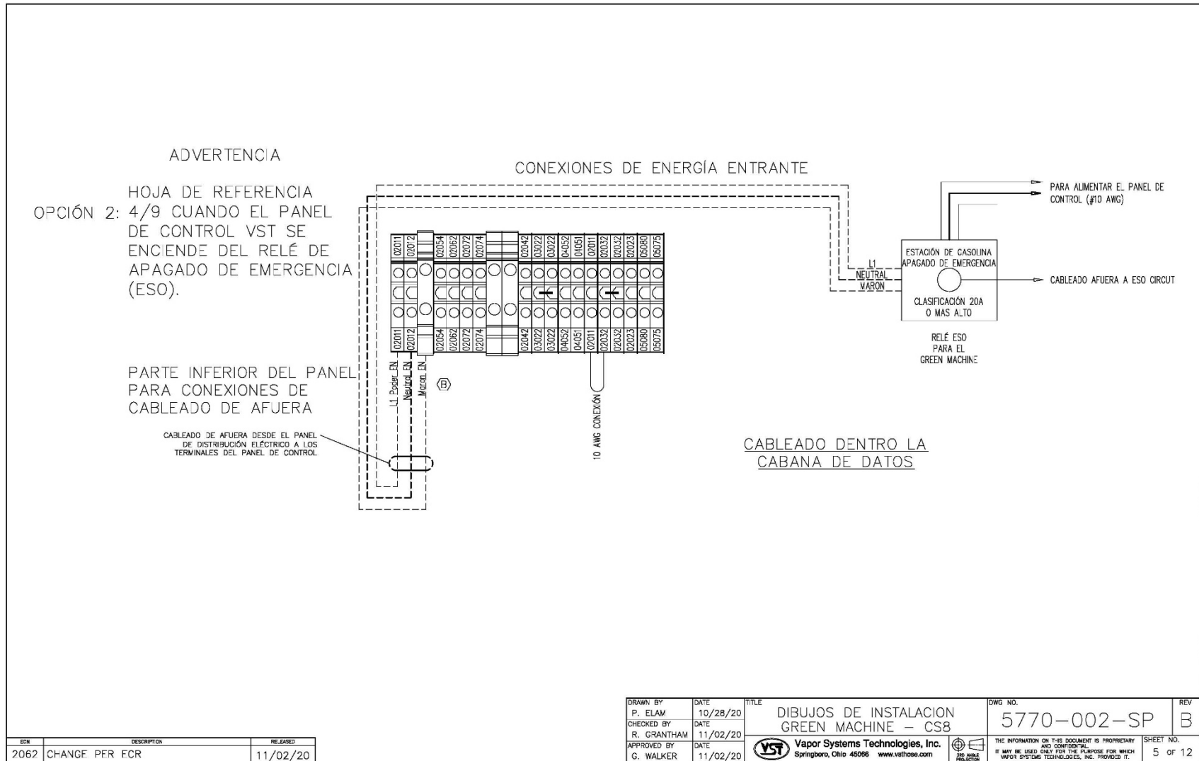
Figura: 3.6 Conexiones de energía del panel de control de VST - Opción 2
