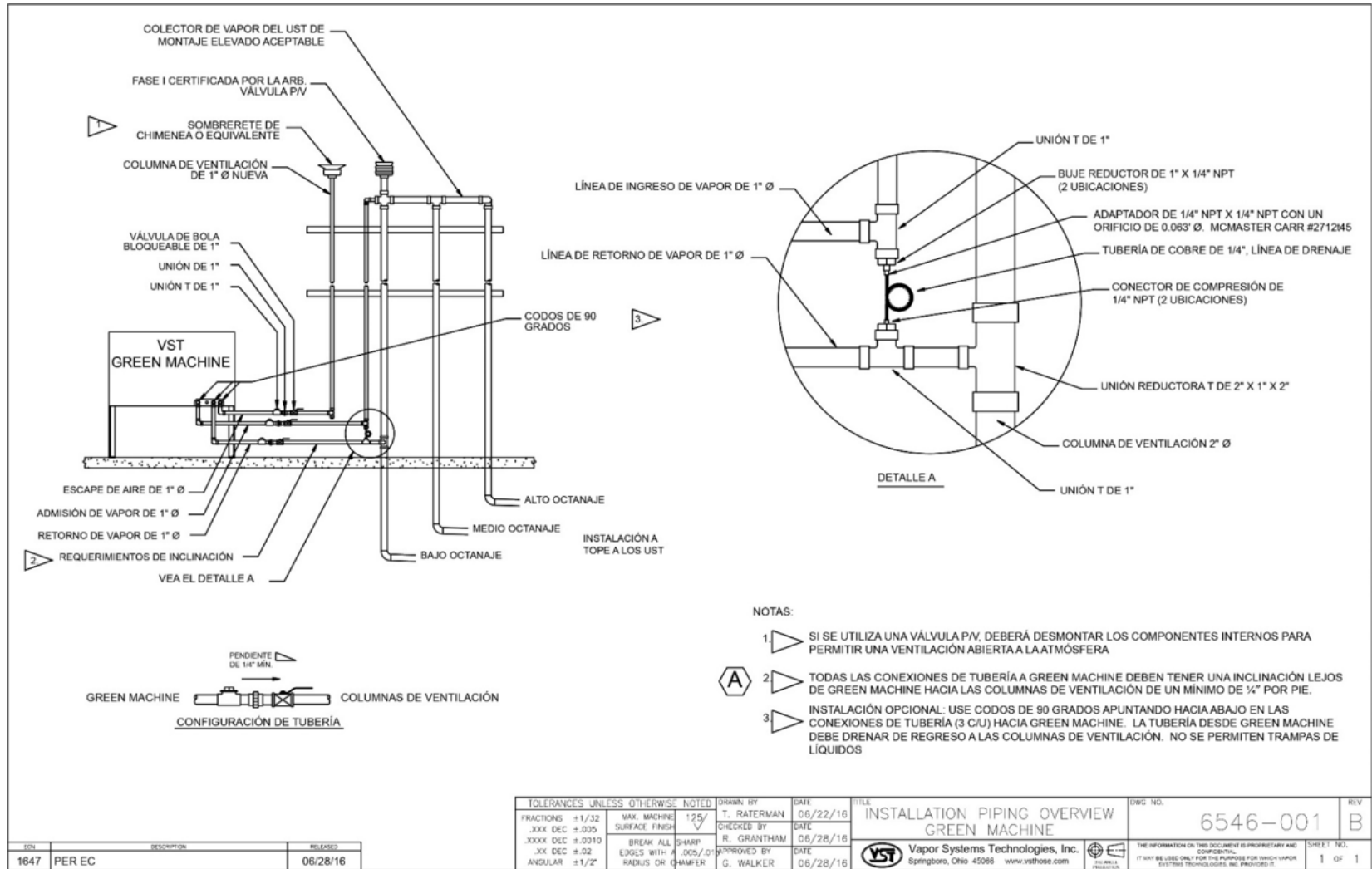
Figura: 1.6 Ejemplo de un GREEN MACHINE con el diseño de la tubería de vapor
