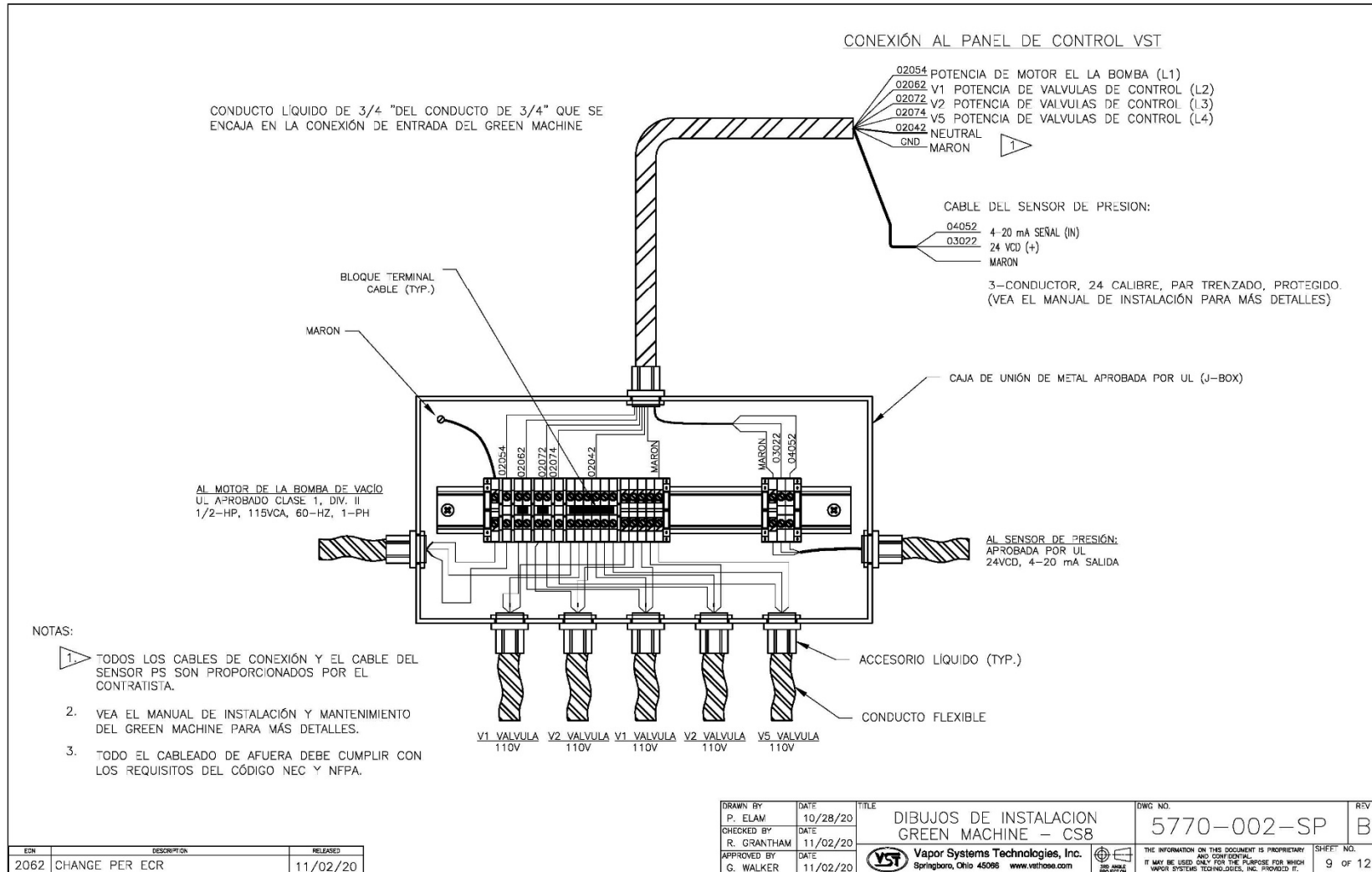
Figura: 3.10 Cableado de campo de la caja de conexiones internas del GREEN MACHINE
