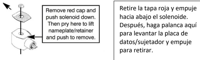
Figura: 9.27 Cómo retirar el tapón rojo de la base del solenoide
