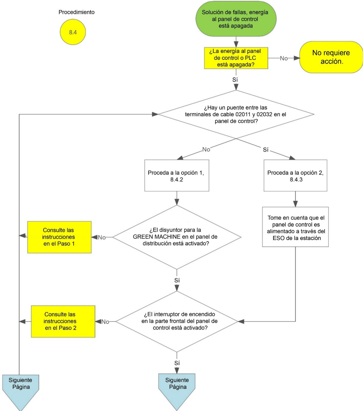
Figura 8-4: La alimentación al panel de control de VST o el controlador de PLC está desconectada
