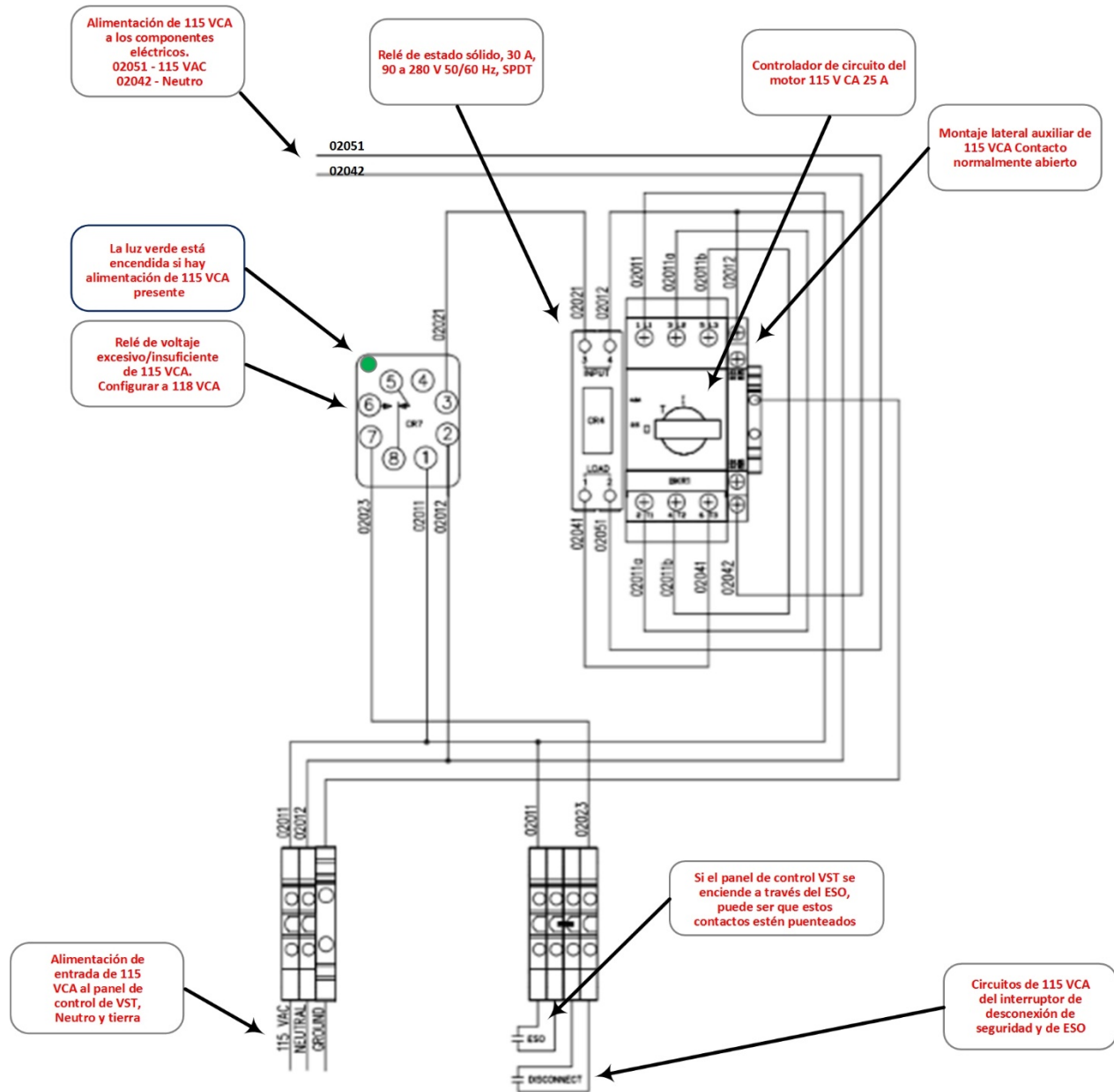
Circuito de alimentación del panel de control de VST, 5-3-2018
