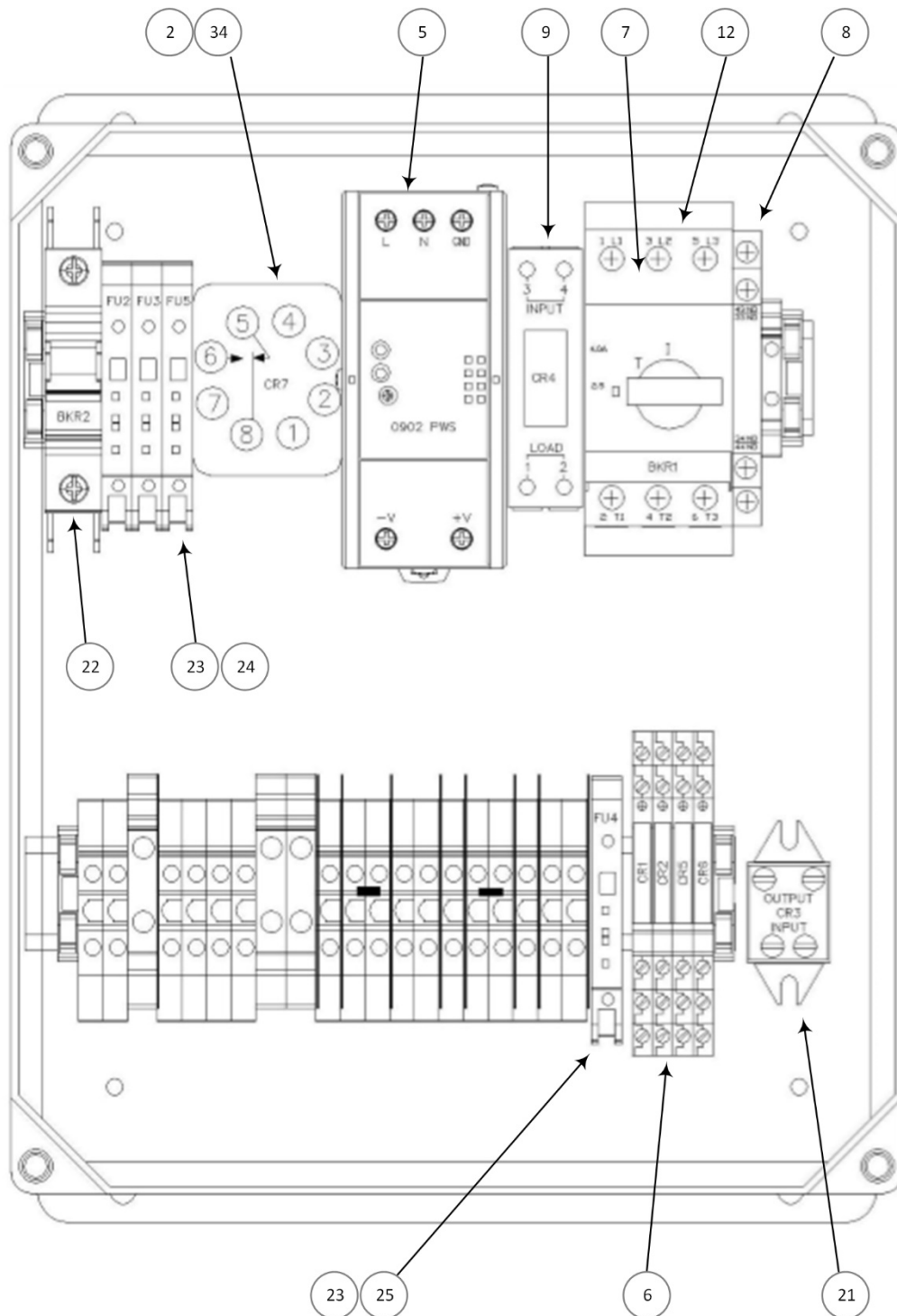
Etiquetas de las piezas internas del panel de control, 20-6-2016
