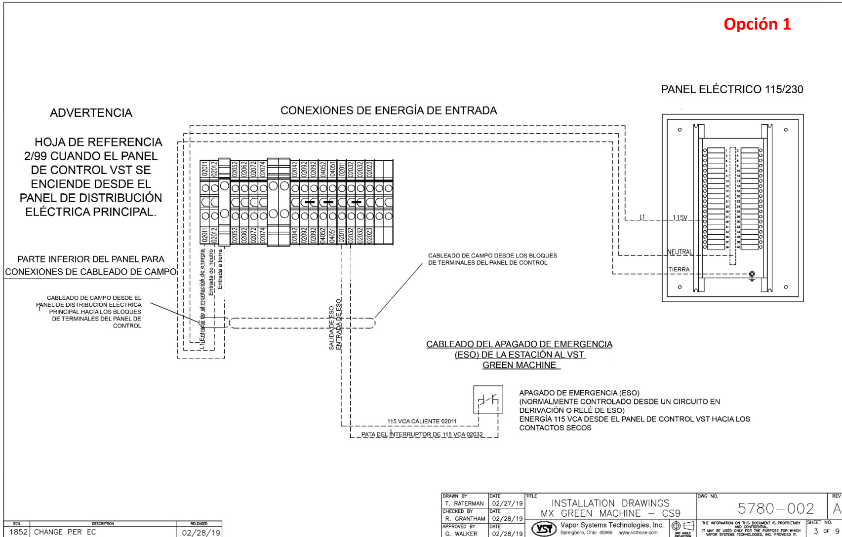
Figura 8-6: Conexiones entrantes de energía
