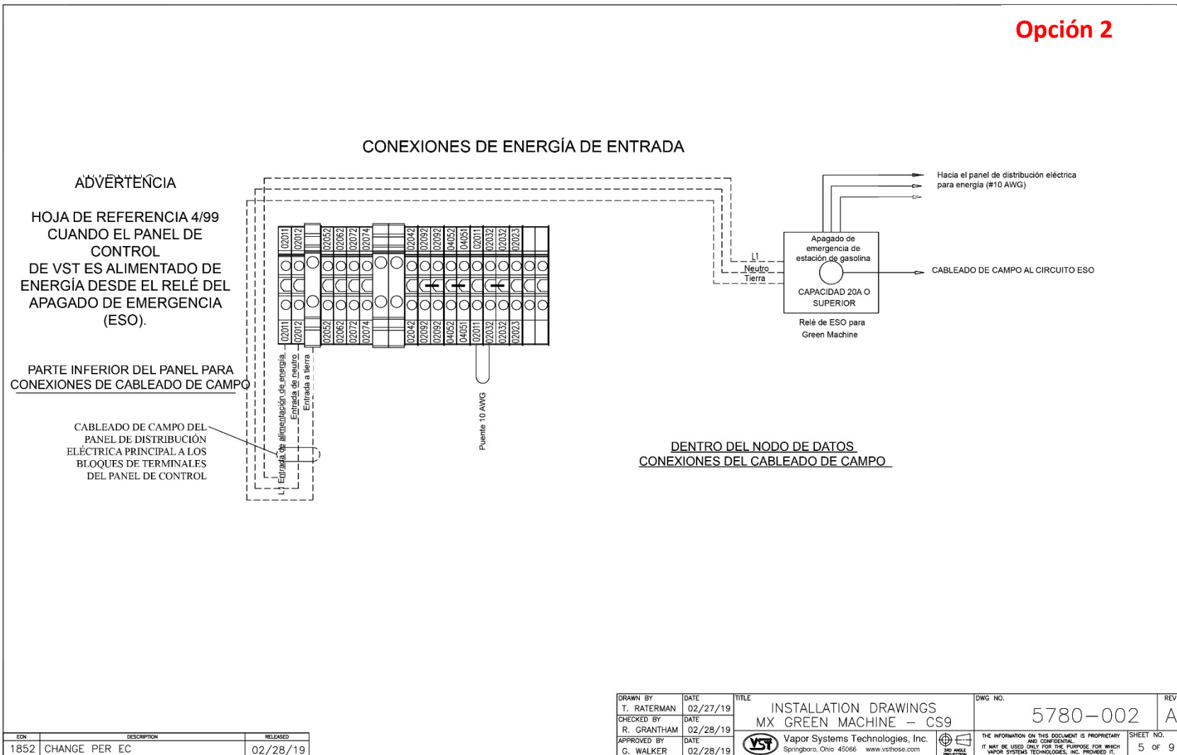
Figura 8-8: Plano de la instalación eléctrica
