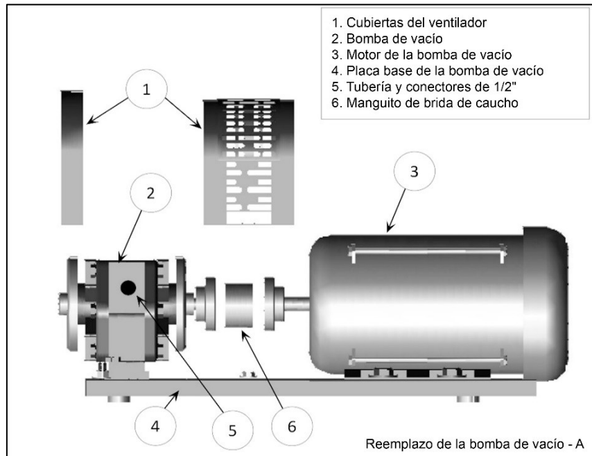
Figura 9-16: Componentes de la bomba de vacío
